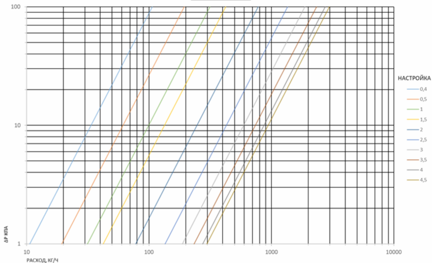
РБК-С Dn15
