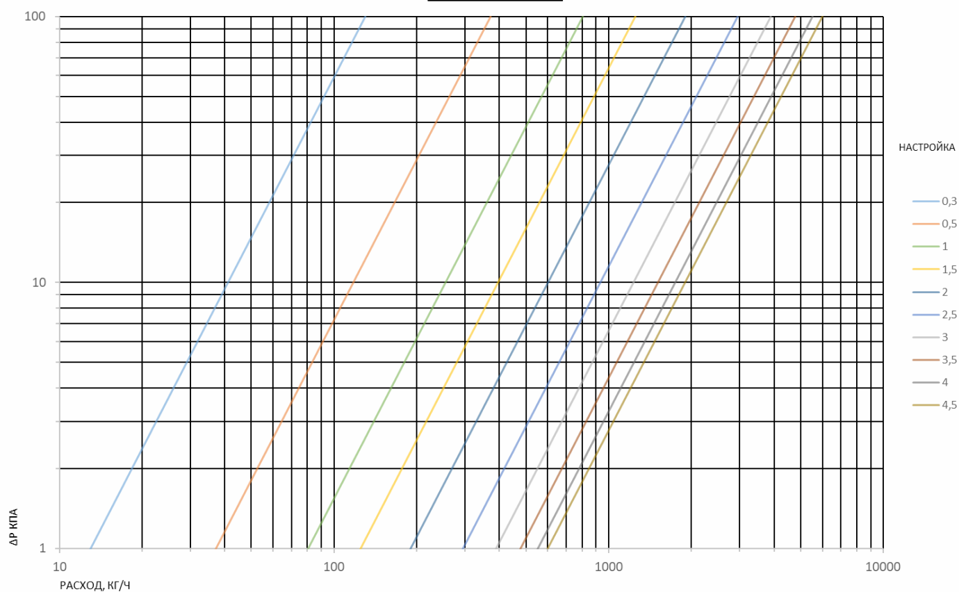
РБК-С Dn 20
